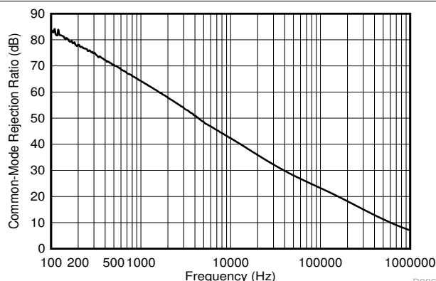
図 5-39. 同相除去比
