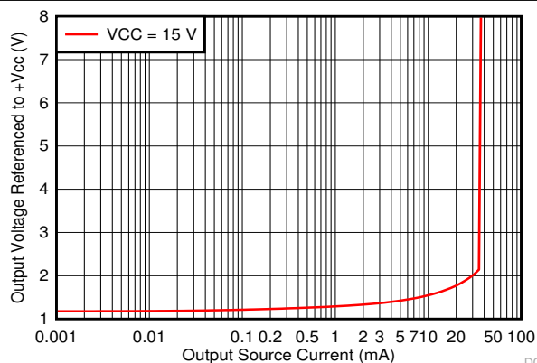
図 5-36. 出力ソース特性
