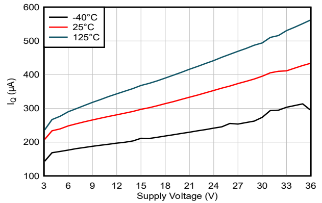
図 5-18. 静止電流と電源電圧との関係
