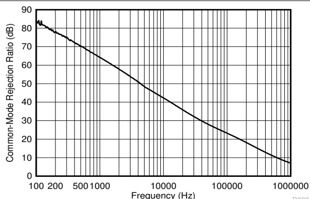
図 5-39. 同相除去比
