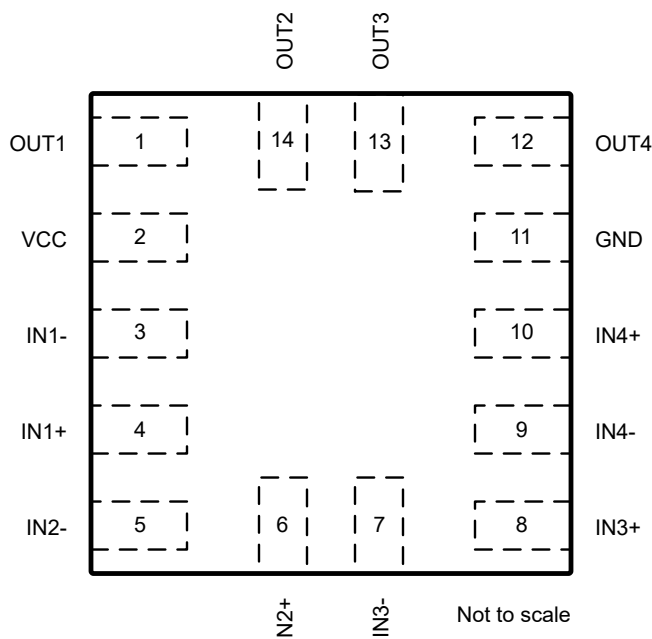
図 4-3. RUC Package 14-Pad X2QFN Top View
