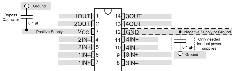
図 8-4. LMx39 Layout Example
