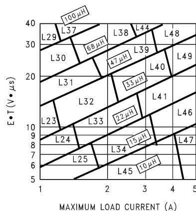
図 7-5. LM2678 - 可変
