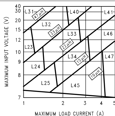
図 7-3. LM2678-5
