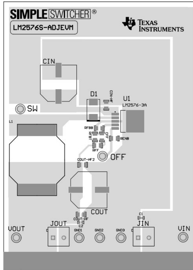
図 8-11. LM2576xx Layout Example
