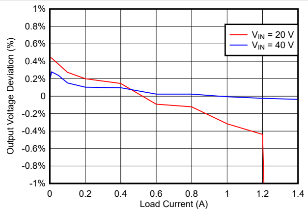
図 8-3. Load Regulation
