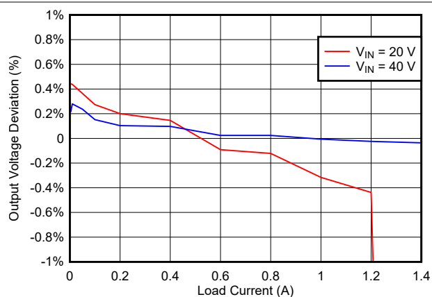
図 6-2. Output Voltage versus Load
