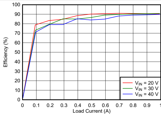
図 8-2. Efficiency
