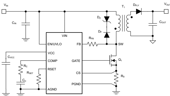
概略回路図
