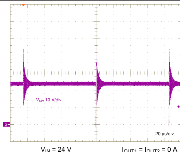
图 8-22. Switch Voltage, No Load
