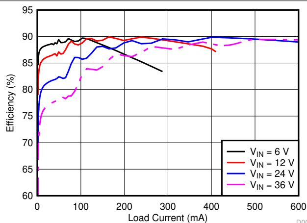
图 8-17. Efficiency (Linear Scale)
