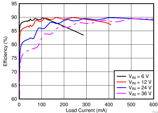
8-17. Efficiency (Linear Scale)
