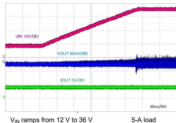
図 9-9. Line Transient
