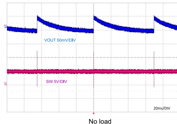
図 9-8. PFM Switching
