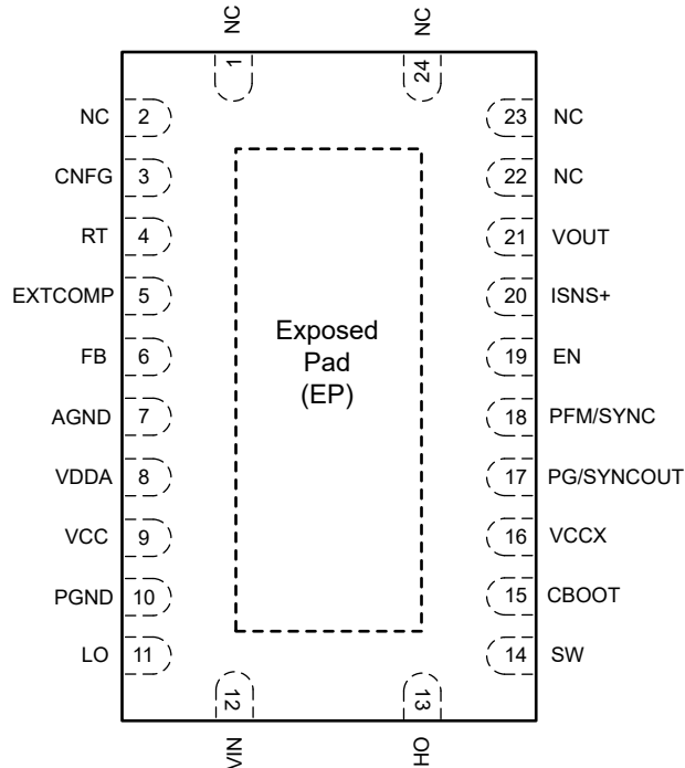
図 6-1. (Top View)
