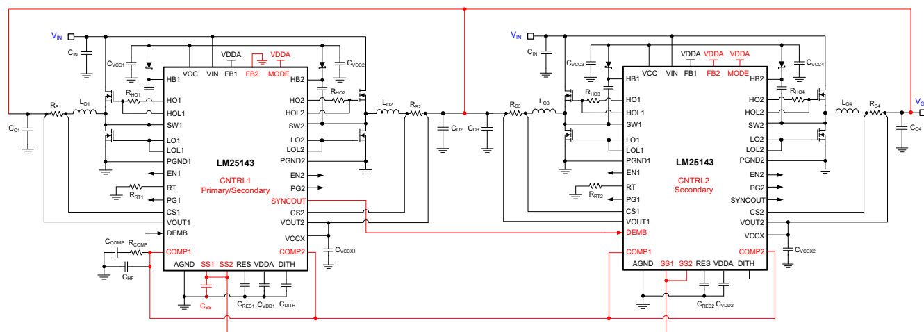
図 9-10. 単一出力インターリーブ動作用に構成された多相レギュレータの回路図
