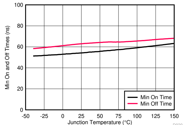
図 8-24. 最小オン時間およびオフ時間 (HO1) と温度との関係
