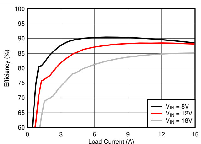
図 10-23. 効率と I_{OUT} との関係、3.3V 出力
