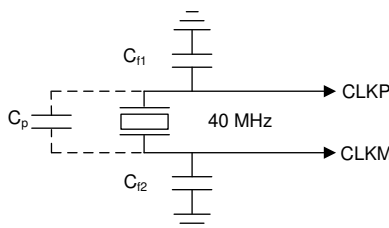
図 7-8. Crystal Implementation
