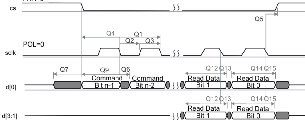
図 7-18. QSPI 読み出し (クロック モード 0)
