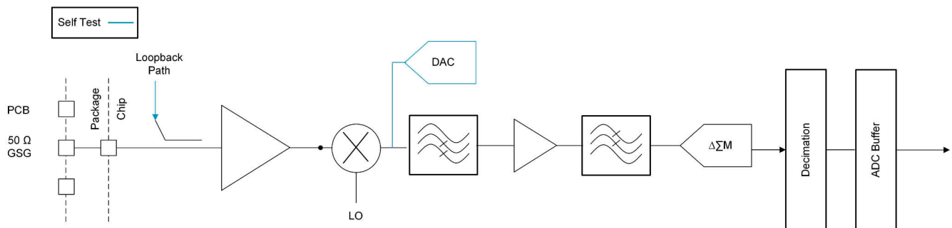
図 8-4. 受信サブシステム (チャンネルごと)
