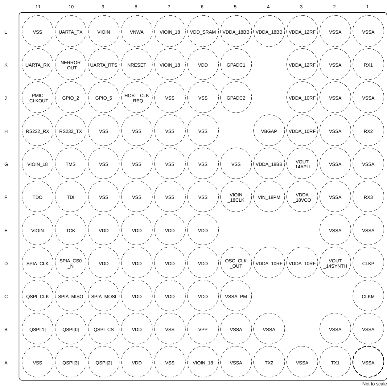
図 6-1. WCSP のピン配置図 (上面図)
