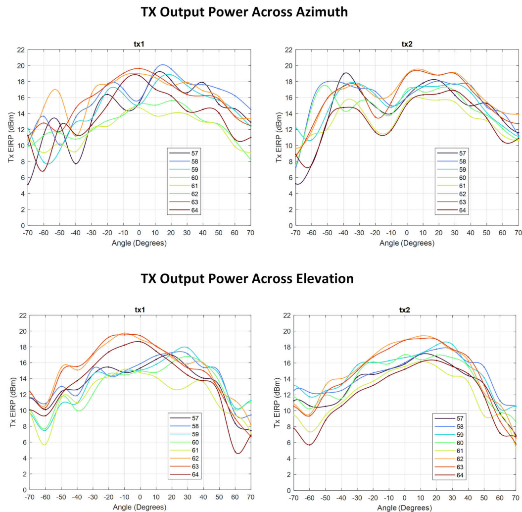
図 7-9. トランスミッタのアンテナ放射パターン
