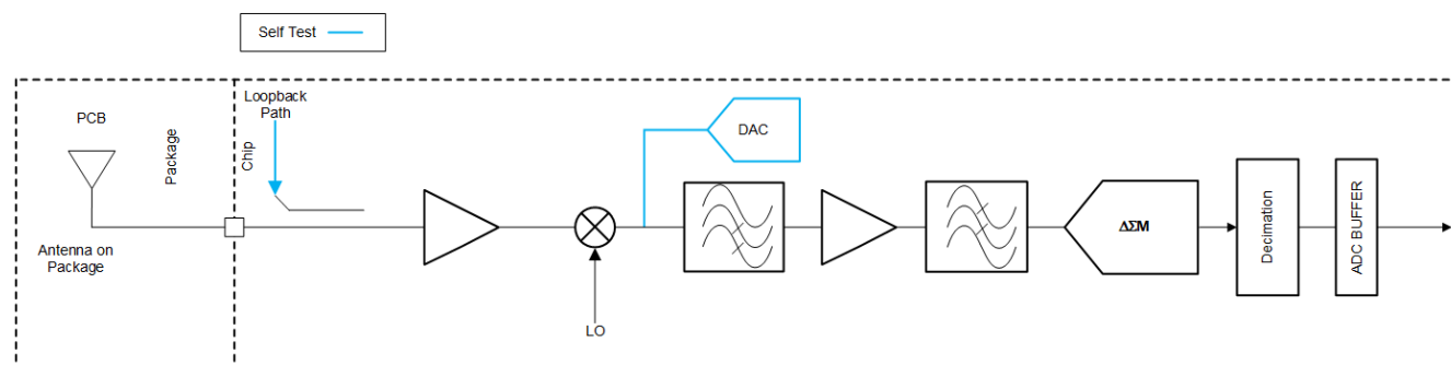
図 8-3. 受信サブシステム (チャンネルごと)
