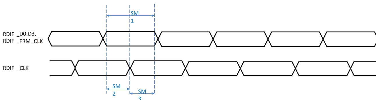
図 7-18. RDIF のタイミング要件
