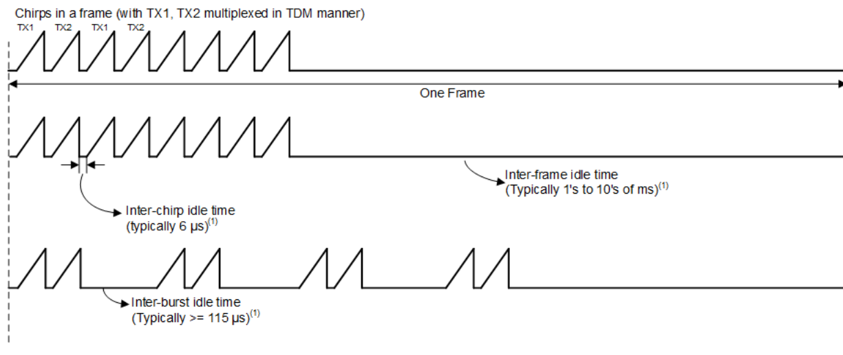
図 7-6. タイミング エンジンがサポートしているチャープ プロファイル
