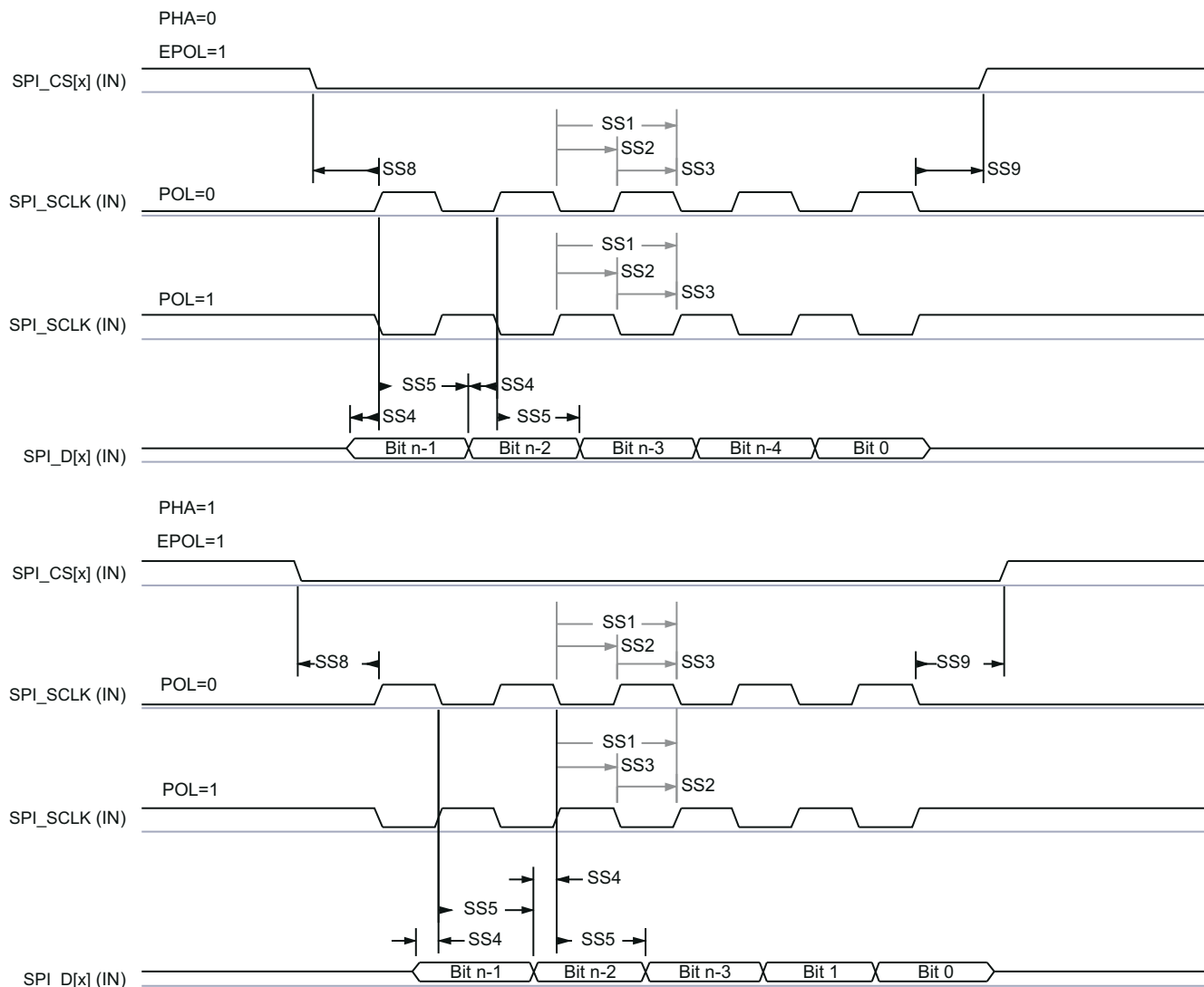
図 7-16. SPI のタイミング - ペリフェラル モードの受信
