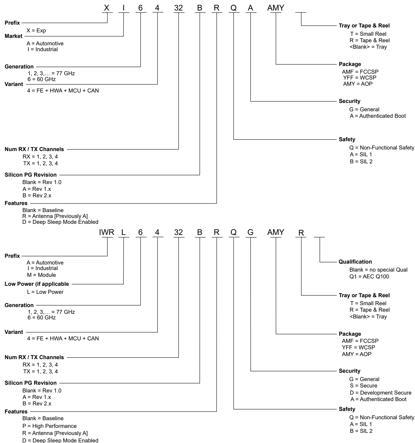
図 10-1. デバイスの命名規則
