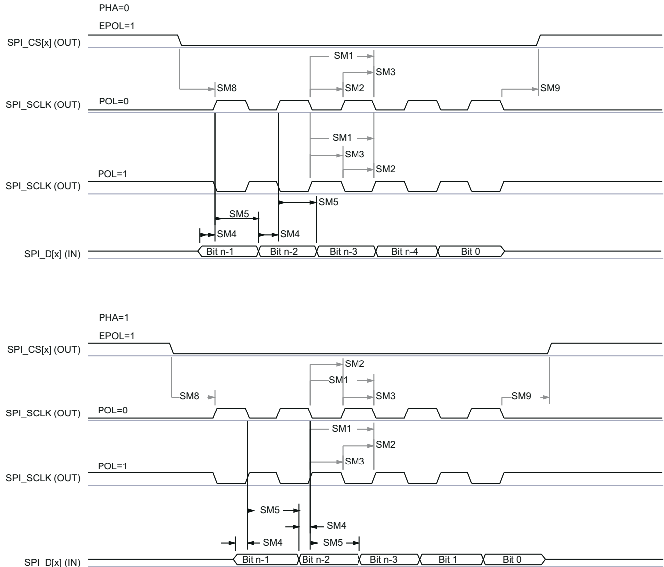
図 7-14. SPI のタイミング - コントローラ モードの受信
