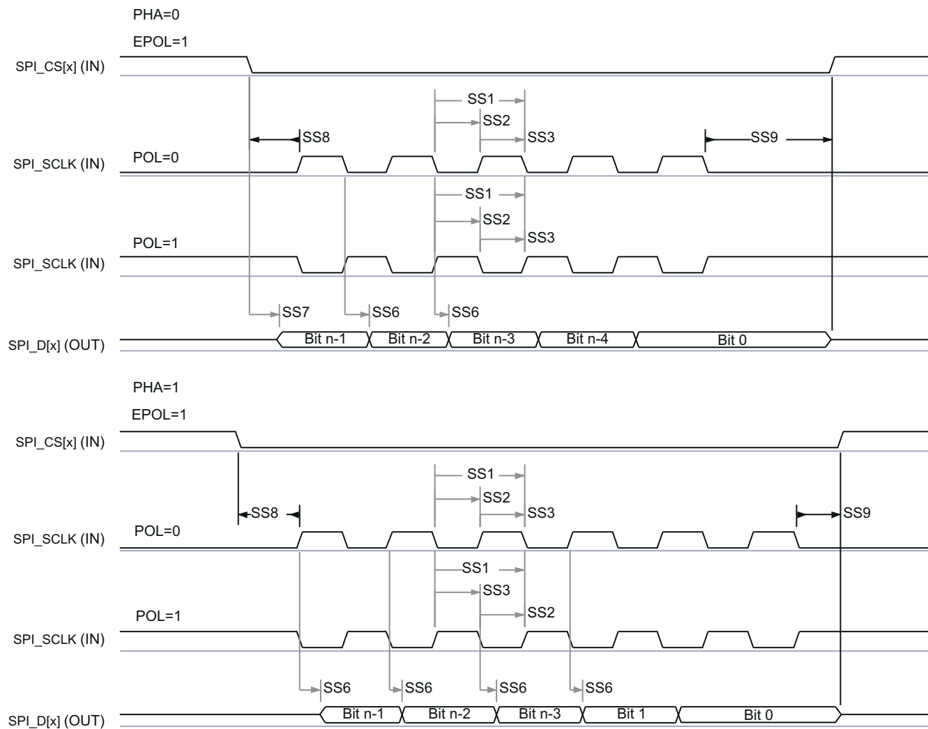
図 7-17. SPI のタイミング - ペリフェラル モードの送信
