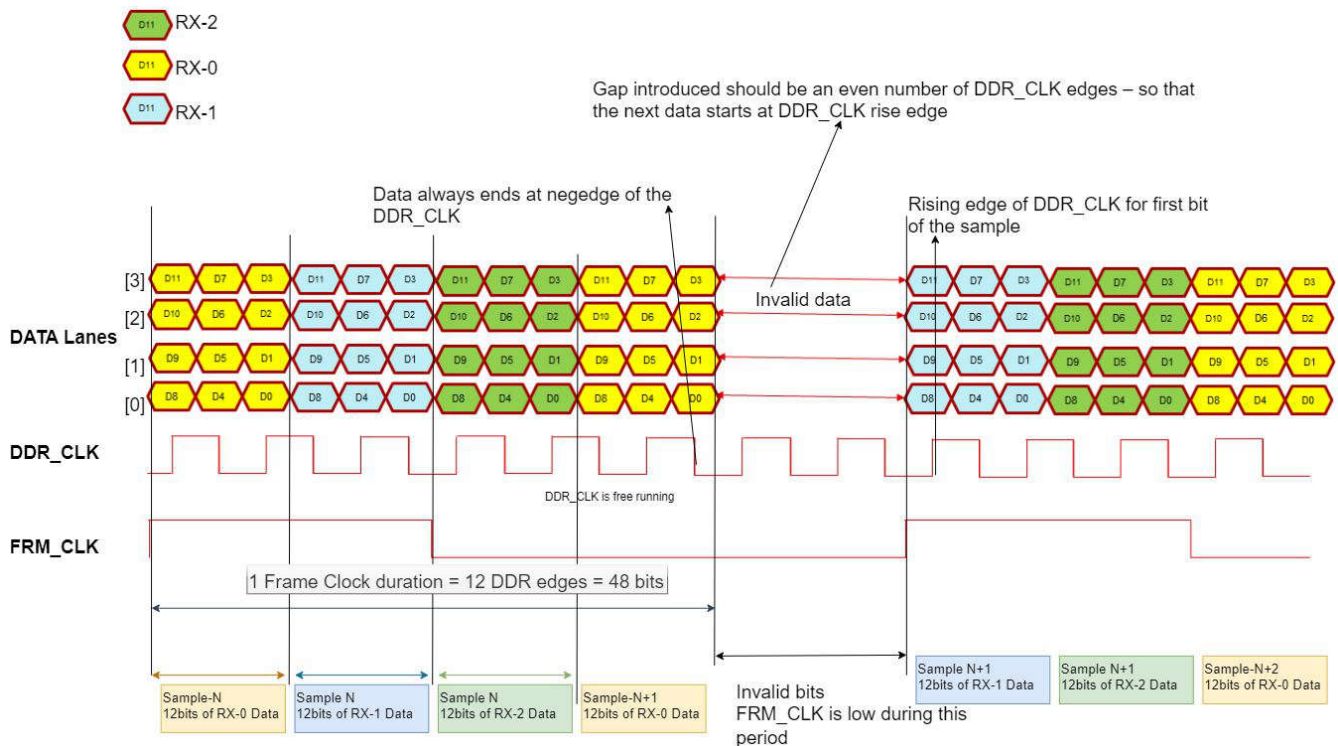
図 7-19. RDIF データ形式
