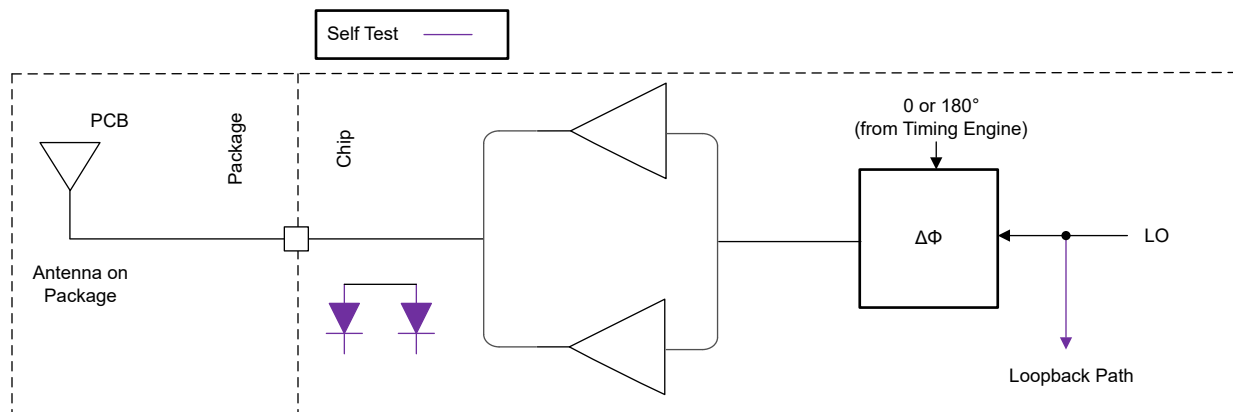
図 8-2. 送信サブシステム (チャンネルごと)
