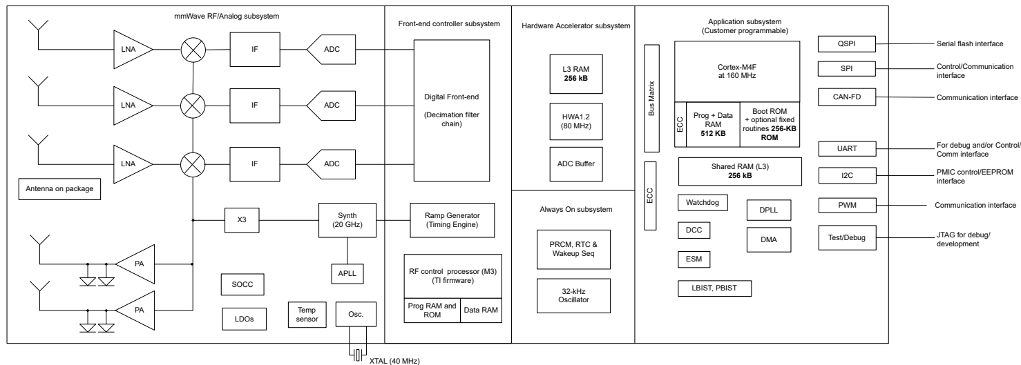
図 4-1. 機能ブロック図
