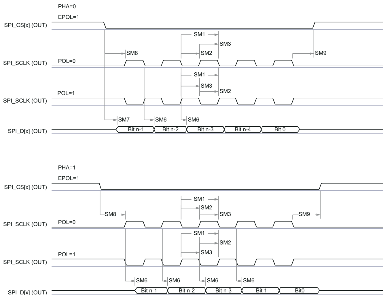
図 7-15. SPI のタイミング - コントローラ モードの送信
