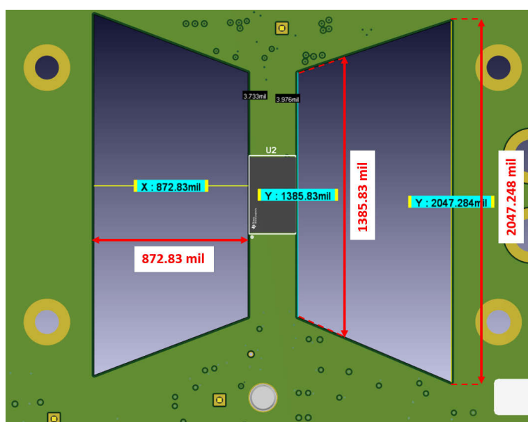
図 7-7. 台形カットアウトと PCB エッジが 0.3mm 未満の大型フォーム ファクタの基板
