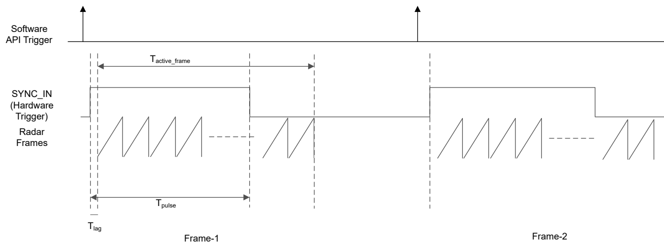
図 7-12. 同期入力ハードウェア トリガ
