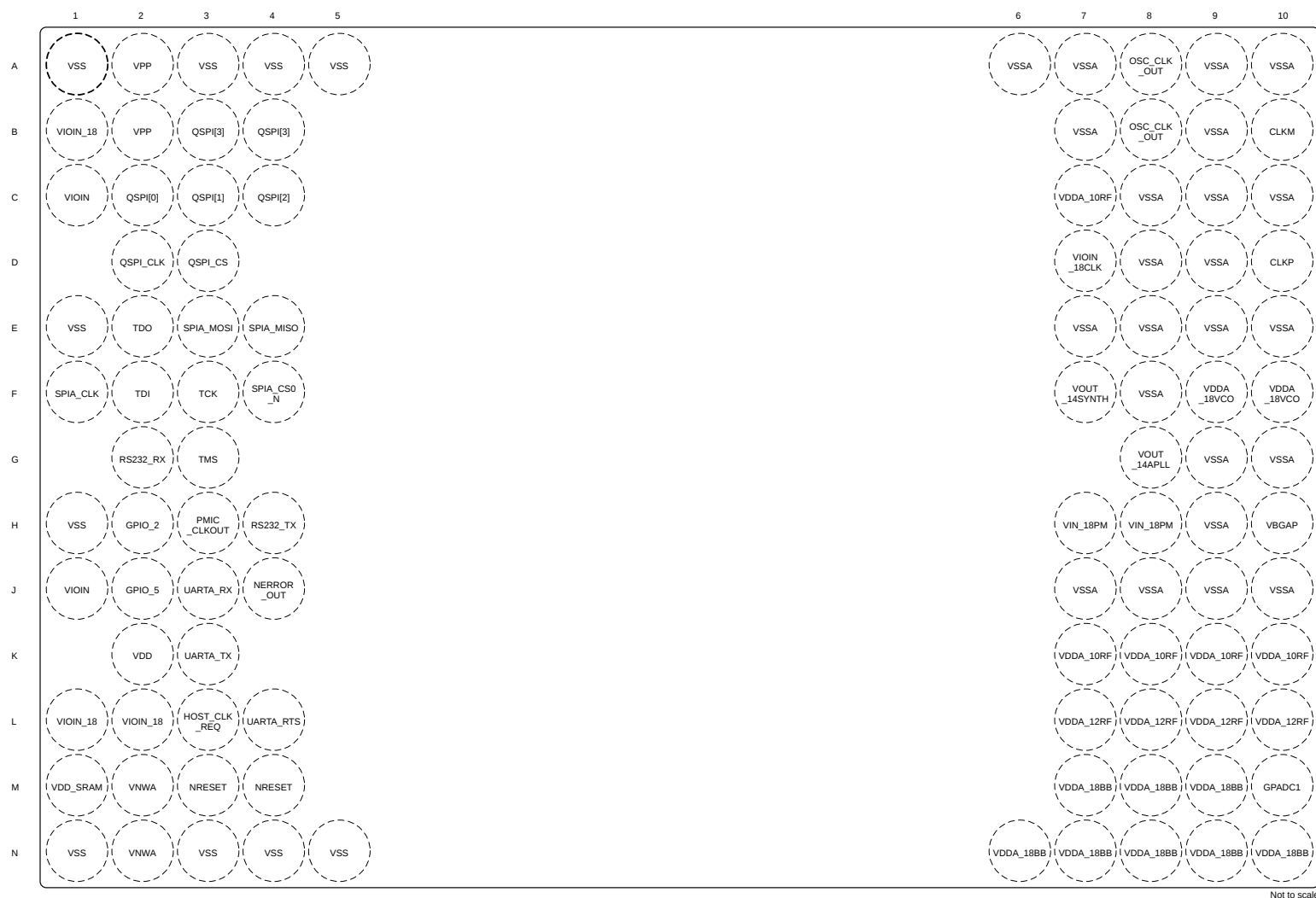
図 6-1. ピン配置図 (上面図)
