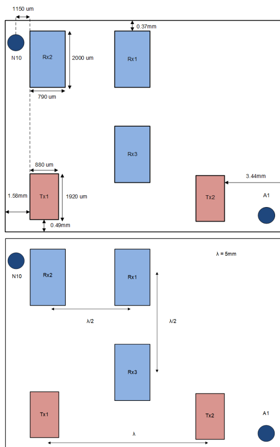
図 7-10. アンテナ位置 (配置と相対間隔)
