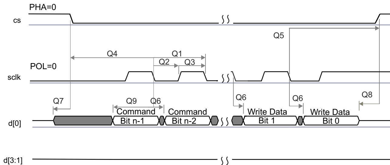
図 7-22. QSPI 書き込み (クロック モード 0)
