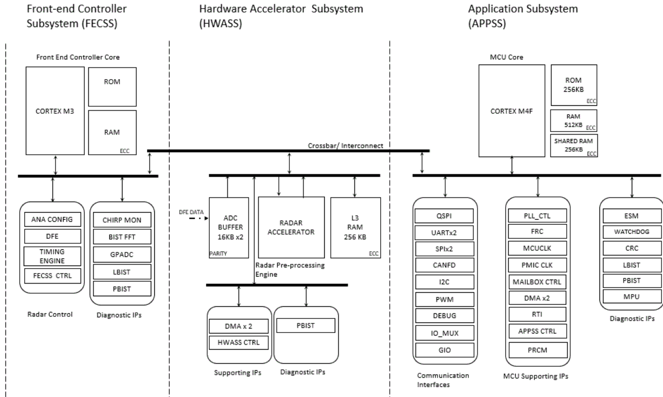
図 8-4. プロセッサ サブシステム
