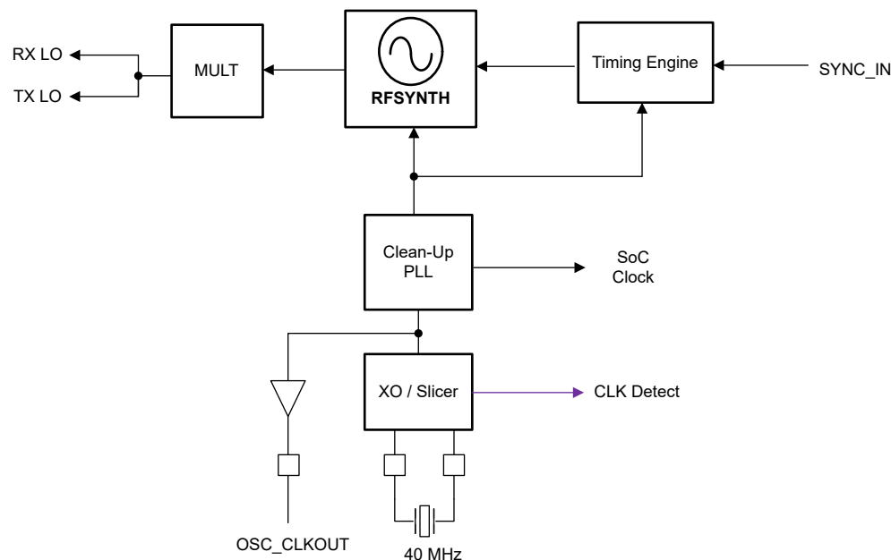
図 8-1. クロック サブシステム
