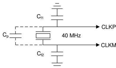
図 7-10. Crystal Implementation
