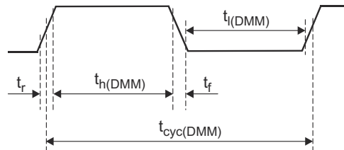
図 7-21. DMMCLK のタイミング
