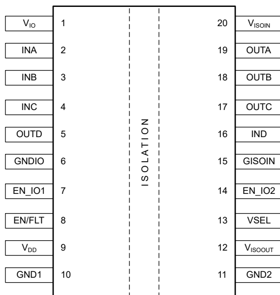
6-2. ISOW7741 DFM Package 20-Pin SOIC-WB Top View
