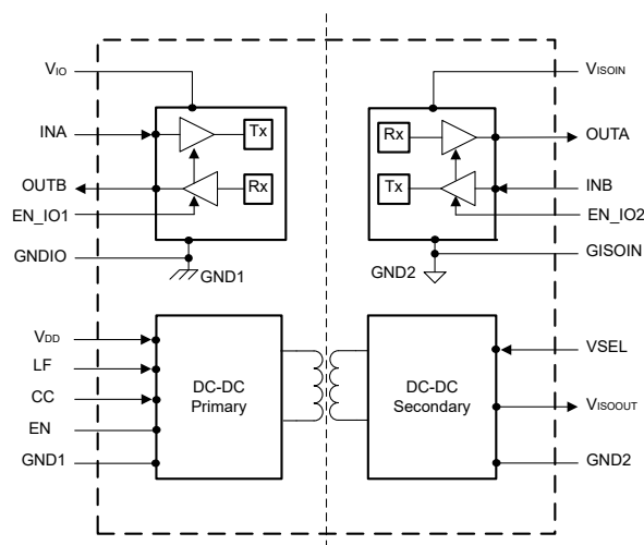
ISOW7721 の概略回路図
