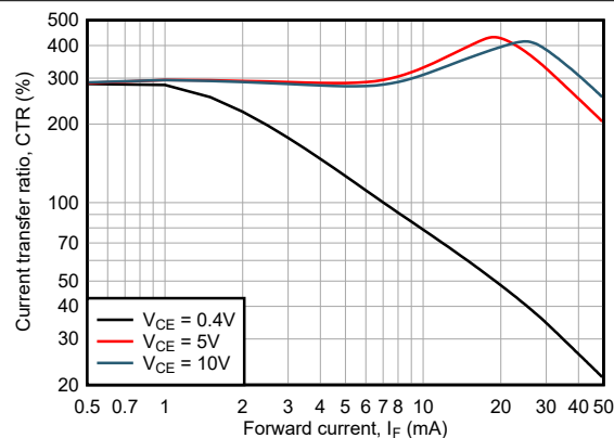
ISOM8112-Q1 & ISOM8117-Q1 T_A = 25^\circ C
