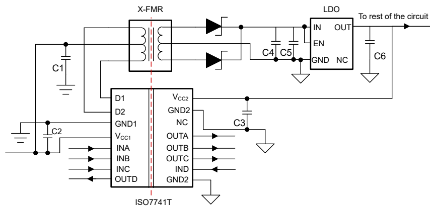
概略回路図
