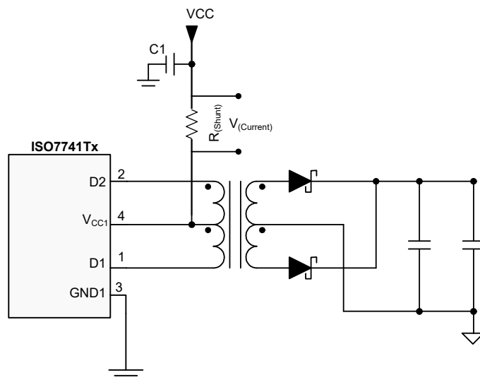
図 6-7. I(slew) Test Setup
