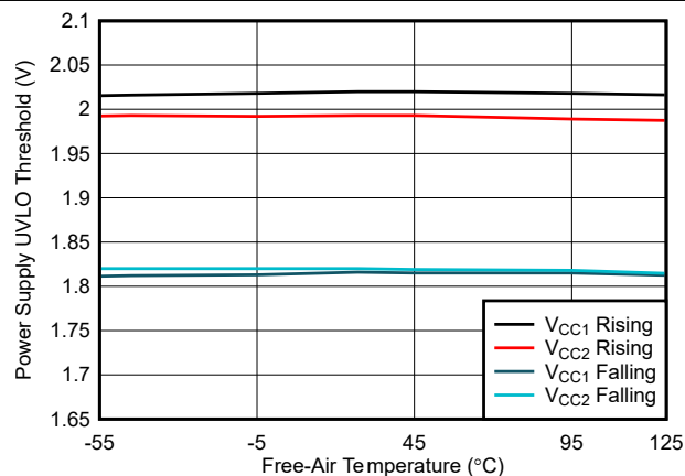
図 5-15. 電源低電圧スレッシュヨルドと周囲温度との関係
