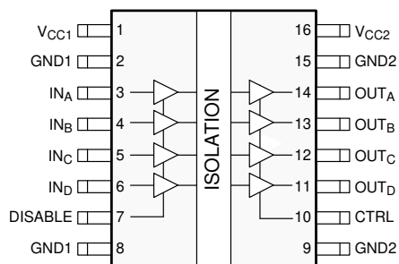
図 4-1. ISO7240CF DW Package 16-Pin SOIC Top View
