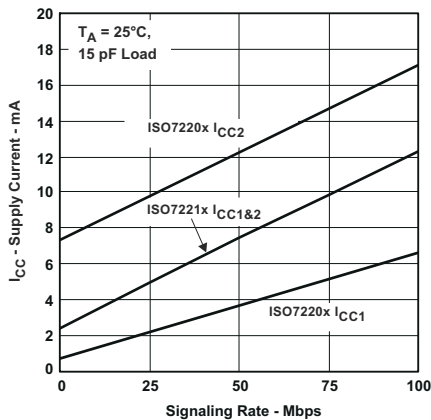
図 5-1. 3.3V RMS 電源電流 対 シグナリング レート (Mbps)
