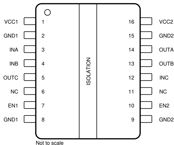
図 5-1. ISO6731-Q1 DW Package 16-Pin SOIC-WB Top View
