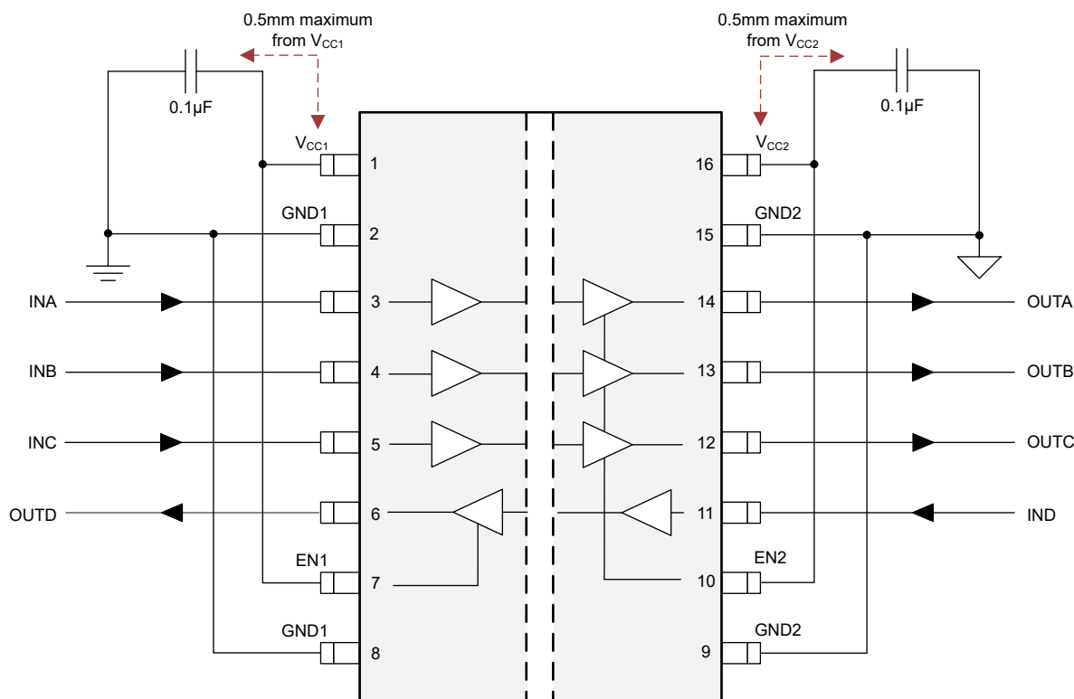
図 8-2. ISO654x の一般的な回路例
