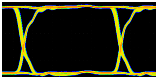
図 9-3. ISO646x アイダイアグラム (100Mbps PRBS 2^{16} - 1 , 5V, 25°C)
