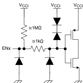
図 7-5. イネーブル (ENx) の回路図
