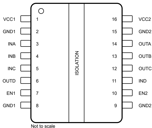
図 4-1. ISO6441 および ISO6441F の上面図
