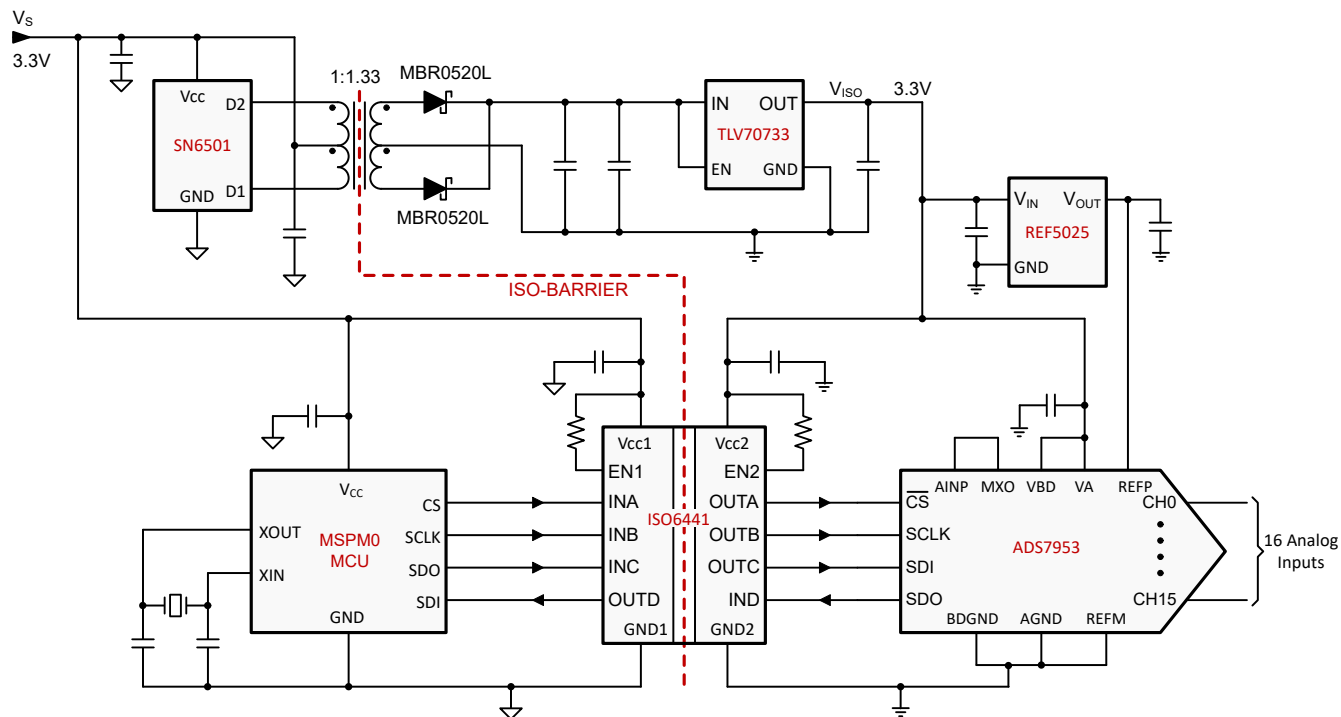
図 8-1. 16 入力のアナログ入力モジュール向け絶縁型 SPI
