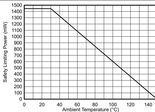
図 5-2. ワイド SOIC (DW-16) パッケージでの安全限界電力の熱特性低下曲線
