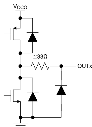
図 7-6. 出力 (OUTx) の回路図
