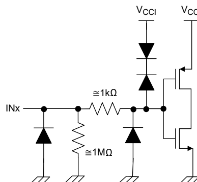
図 7-4. 入力 (INx) がデフォルトが Low (接尾辞 F が付いたデバイス) の回路図
