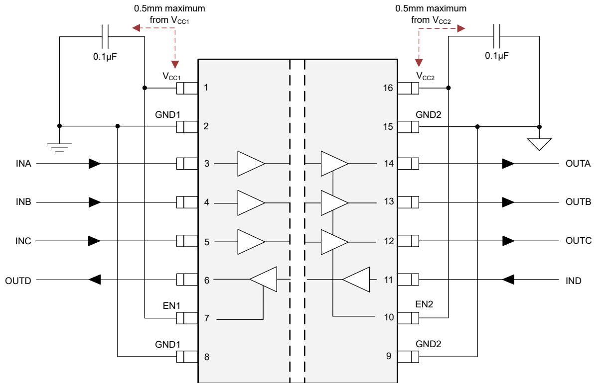
図 8-2. ISO644x の一般的な回路例
