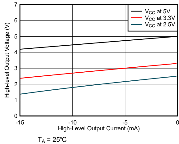
図 5-5. High レベル出力電圧と High レベル出力電流との関係
