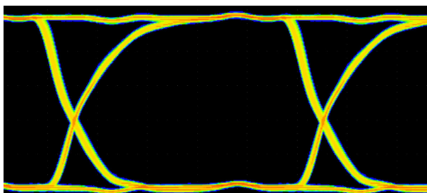
図 8-3. ISO644x アイダイアグラム (100Mbps PRBS 2^{16} - 1 、5V、25°C)
