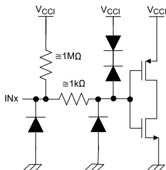
図 7-3. 入力 (INx) がデフォルトが High (接尾辞 F なしのデバイス) の回路図
