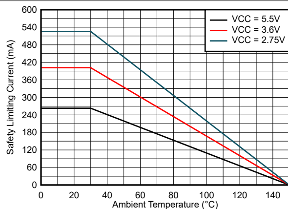
図 5-1. ワイド SOIC (DW-16) パッケージでの安全限界電流の熱特性低下曲線
