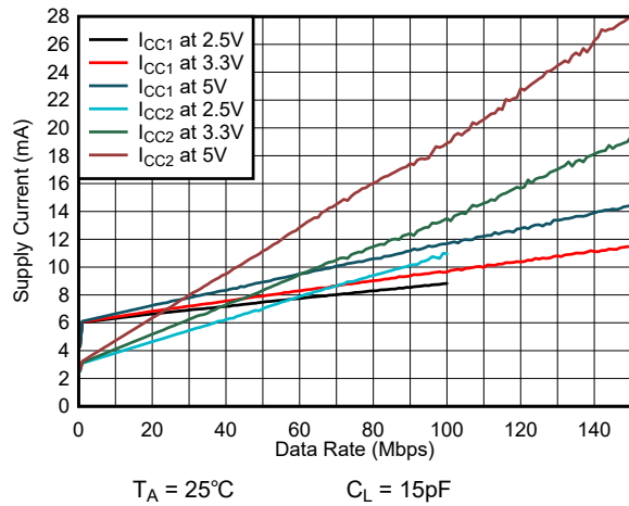
図 5-3. ISO6441 または ISO6441F の消費電流とデータレートとの関係 (15pF 負荷時)
