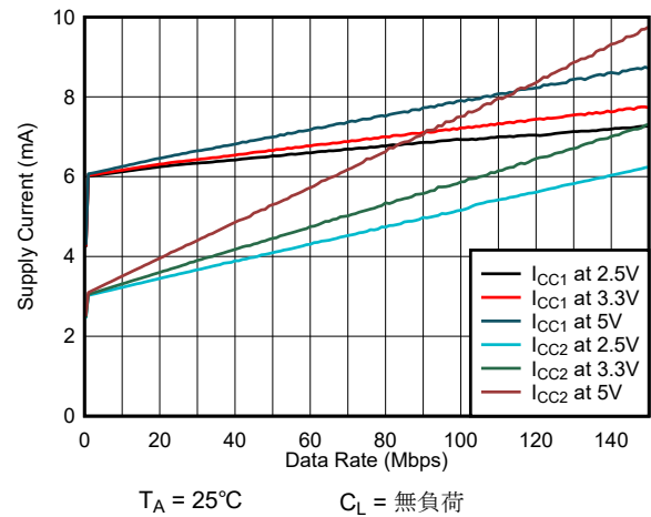
図 5-4. ISO6441 または ISO6441F の消費電流とデータレートとの関係 (無負荷時)
