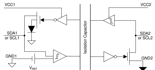
絶縁型双方向データ・チャネルの概略回路図
