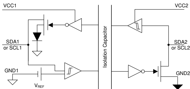
概略回路図
