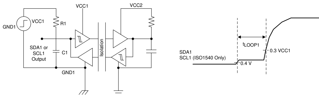
图 7-1. Test Diagram
