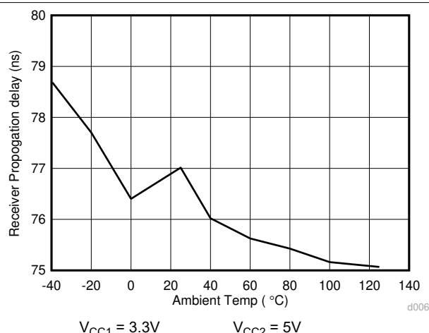
図 7-25. ISO143x レシーバの伝搬遅延 (ns) と温度 ( ^\circ\text{C} ) との関係
