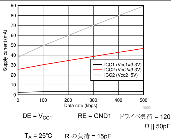
図 7-5. ISO141x の電源電流とデータ レートとの関係 - 120Ω||50pf 負荷
