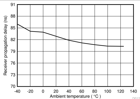
図 7-24. ISO141x レシーバの伝搬遅延 (ns) と温度 ( ^\circ\text{C} ) との関係
