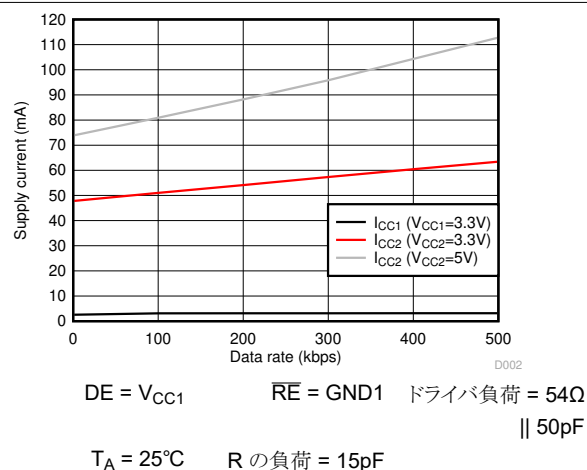
図 7-4. ISO141x の電源電流とデータ レートとの関係 - 54Ω||50pf 負荷
