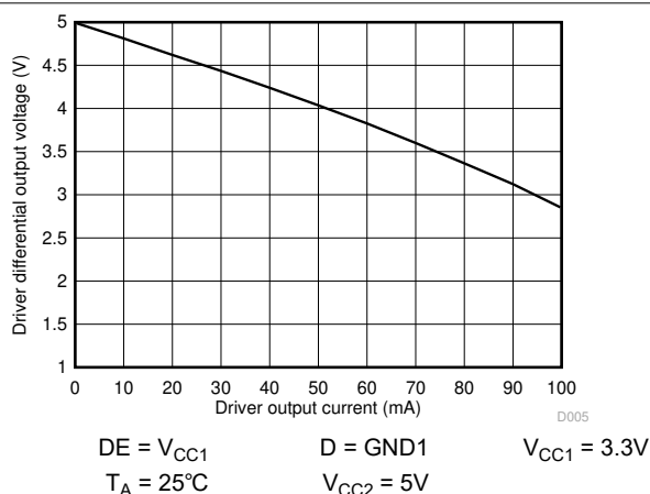
図 7-13. ドライバ差動出力電圧とドライバ出力電流との関係
