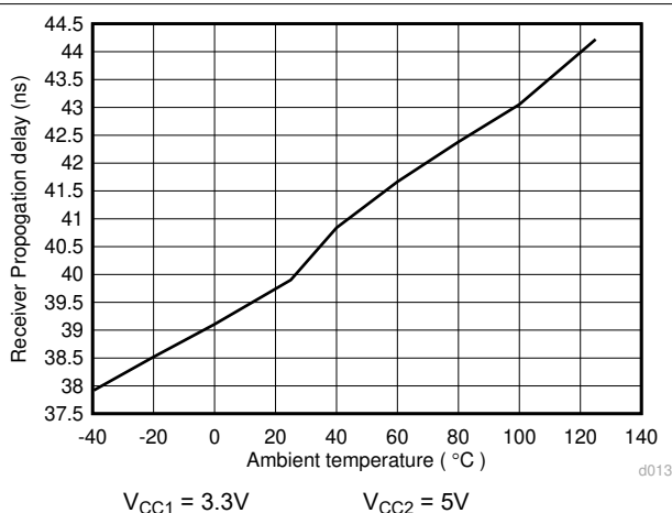
図 7-26. ISO145x レシーバの伝搬遅延 (ns) と温度 ( ^\circ\text{C} ) との関係
