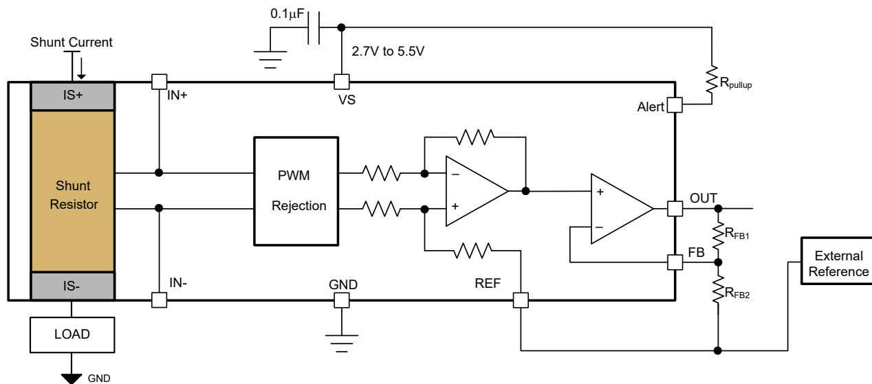
6-10. Thermal Alert Function
