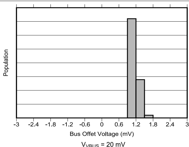
5-9. Bus Input Offset Voltage Production Distribution
