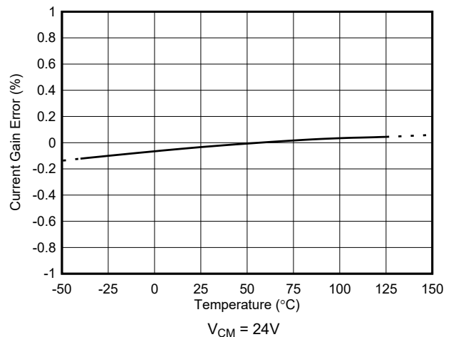
図 5-7. 電流ゲイン誤差と温度との関係
