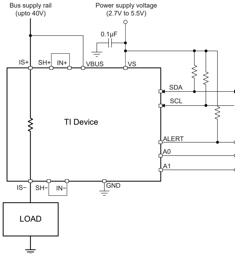
図 8-2. INA745x-Q1 下限側センシング アプリケーション図
