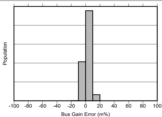
図 5-11. バス入力ゲイン誤差の製造分布 V_{VBUS} = 20\text{mV}
