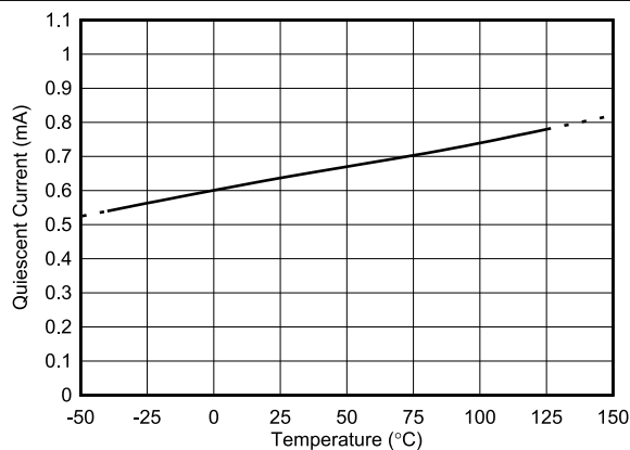
図 5-16. アクティブ I_Q と温度の関係
