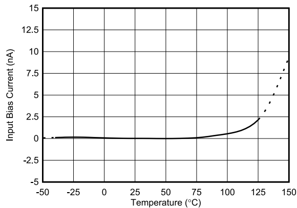
図 5-14. 入力バイアス電流と温度との関係
