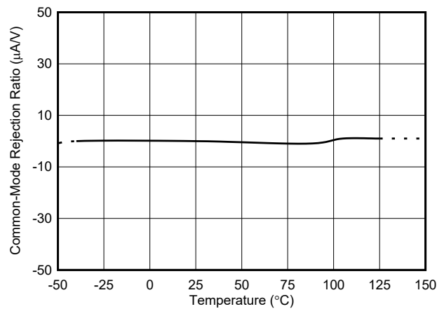
図 5-5. 電流同相除去比と温度との関係
