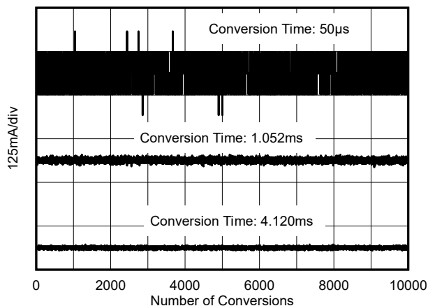
図 6-9. ノイズと変換時間の関係 (平均化 = 1)
