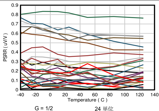
図 7-23. PSRR と温度との関係
