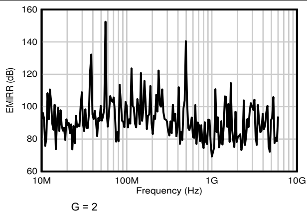
図 7-64. 差動モード EMI 除去比
