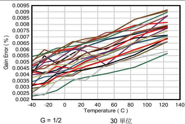
図 7-29. ゲイン誤差と温度との関係
