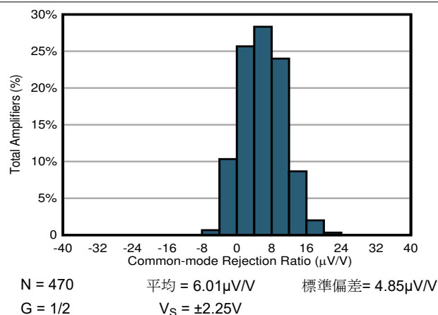
図 7-15. CMRR の標準的な分布
