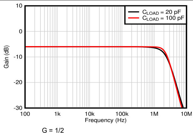
図 7-31. 閉ループ・ゲインと周波数との関係
