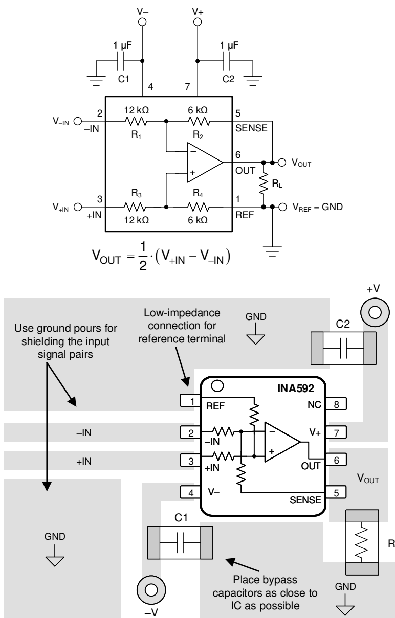
図 11-1. SOIC と VSSOP パッケージの回路図とそれに関連する PCB レイアウトの例
