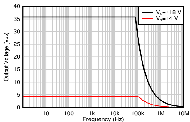
図 7-22. 最大出力電圧と周波数との関係
