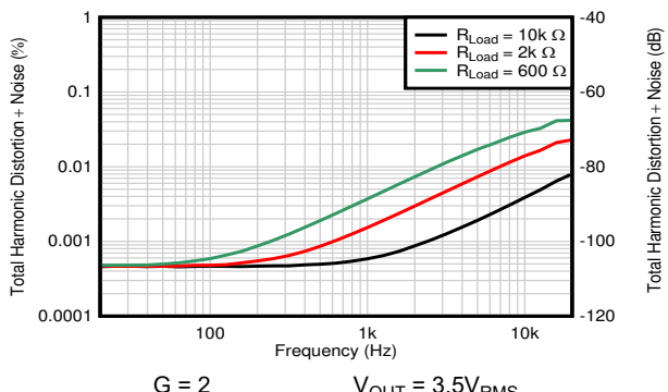
図 7-54. THD+N と周波数との関係
