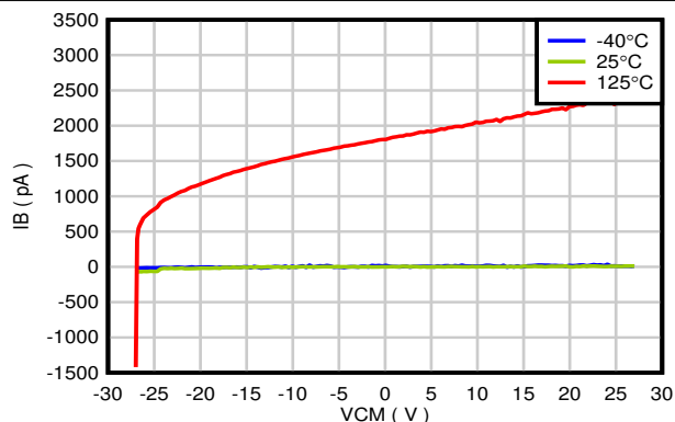
G = 2 図 7-14. 入力バイアス電流と同相電圧との関係
