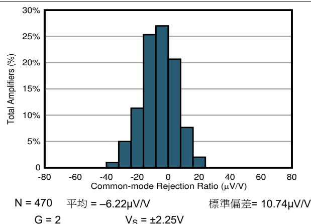
図 7-16. CMRR の標準的な分布
