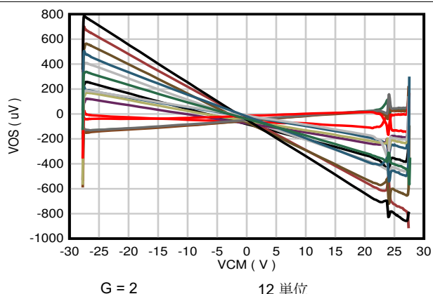
図 7-10. オフセット電圧と同相電圧との関係
