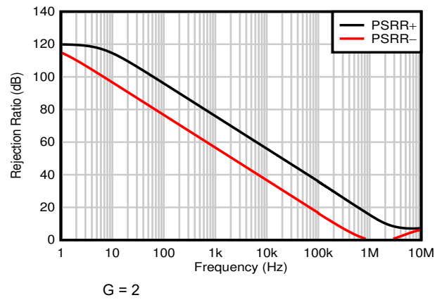
図 7-26. PSRR と周波数との関係 (RTI)
