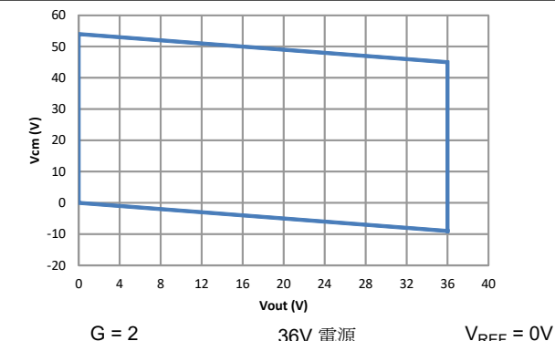
図 7-72. 入力同相電圧と出力電圧との関係
