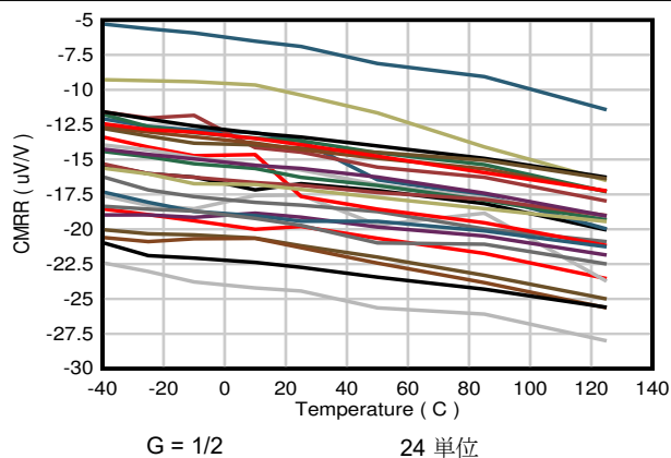
図 7-19. CMRR と温度との関係
