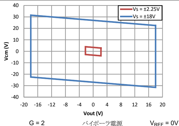
図 7-68. 入力同相電圧と出力電圧との関係
