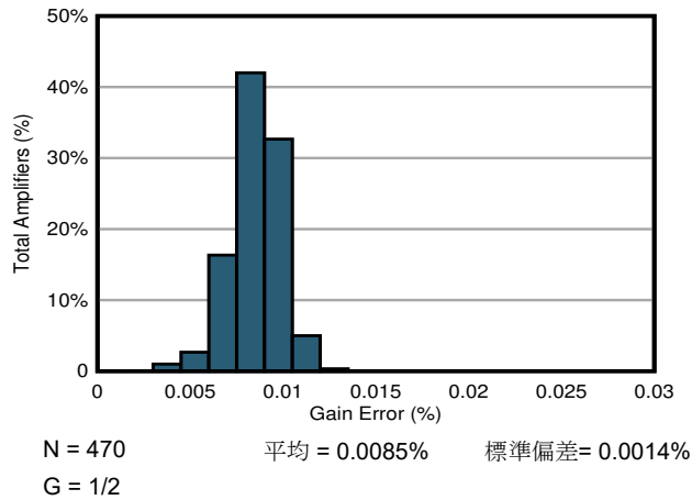
図 7-27. ゲイン誤差の標準的な分布
