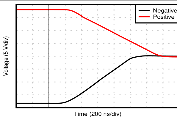
図 7-46. 大信号ステップ応答
