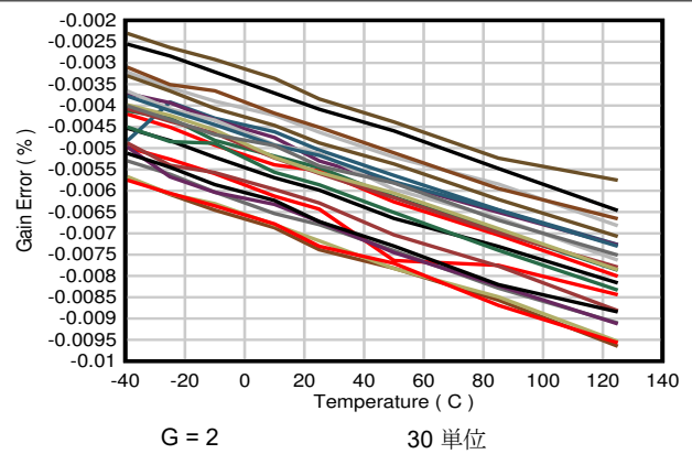
図 7-30. ゲイン誤差と温度との関係
