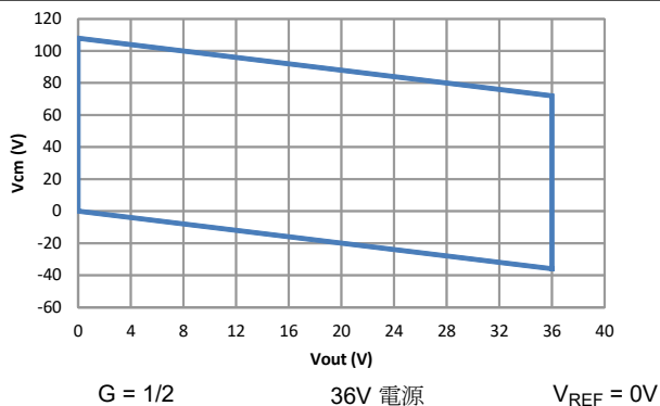
図 7-71. 入力同相電圧と出力電圧との関係
