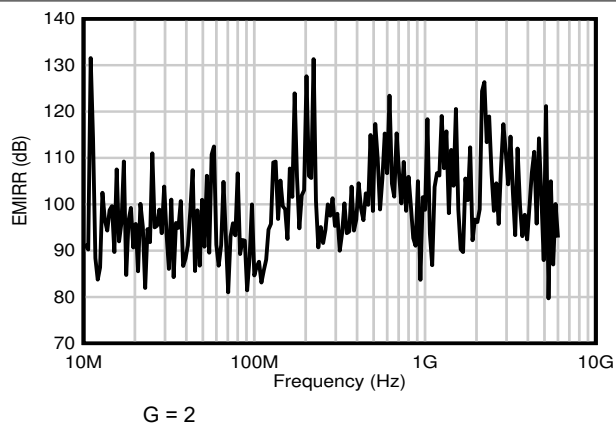
図 7-66. 同相 EMI 除去比
