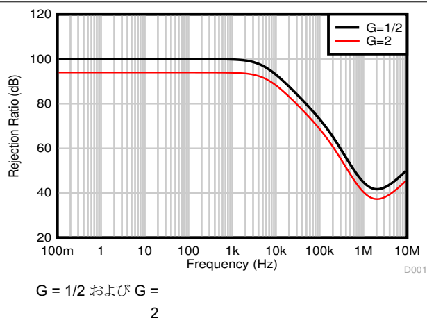
図 7-21. 同相除去比と周波数との関係 (RTI)
