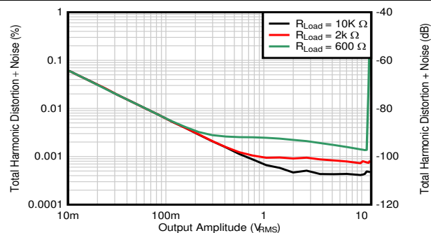
図 7-55. THD+N 比と出力振幅との関係
