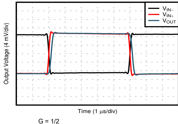
図 7-51. 小信号ステップ応答
