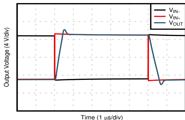
図 7-43. セットリング・タイム
