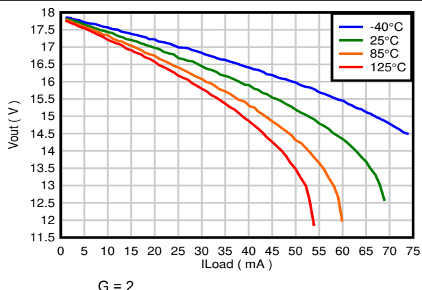
図 7-40. 正出力電圧と出力電流との関係 (ソース)
