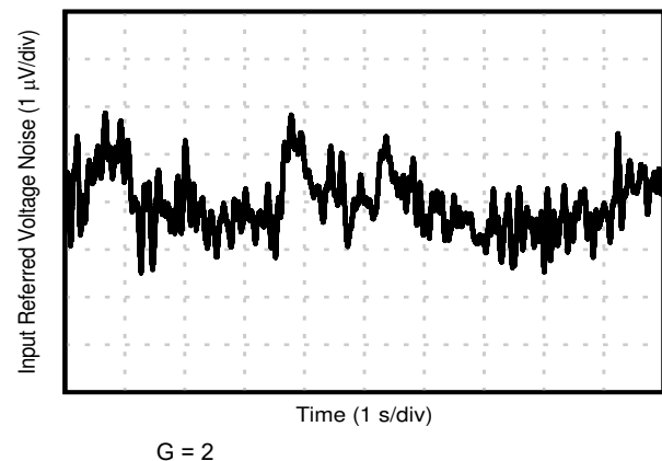
図 7-36. 0.1Hz~10Hz RTI 電圧ノイズ
