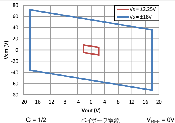
図 7-67. 入力同相電圧と出力電圧との関係
