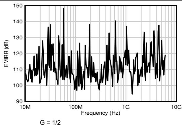
図 7-63. 差動モード EMI 除去比
