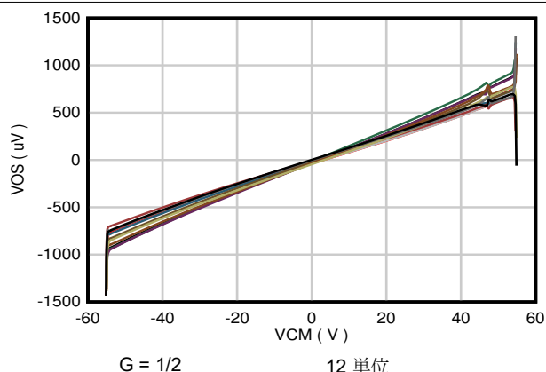
図 7-9. オフセット電圧と同相電圧との関係
