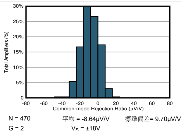
図 7-18. CMRR の標準的な分布
