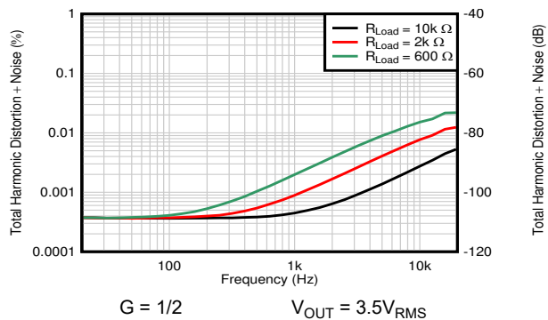
図 7-53. THD+N と周波数との関係
