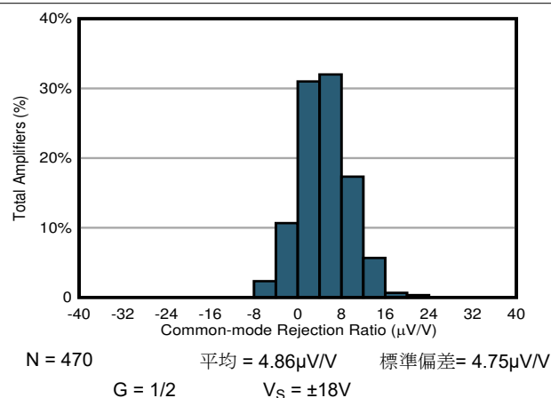
図 7-17. CMRR の標準的な分布
