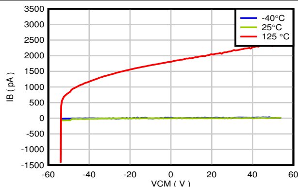
G = 1/2 図 7-13. 入力バイアス電流と同相電圧との関係
