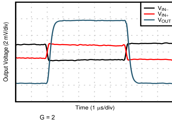
図 7-52. 小信号ステップ応答
