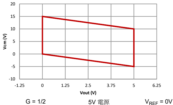
図 7-69. 入力同相電圧と出力電圧との関係
