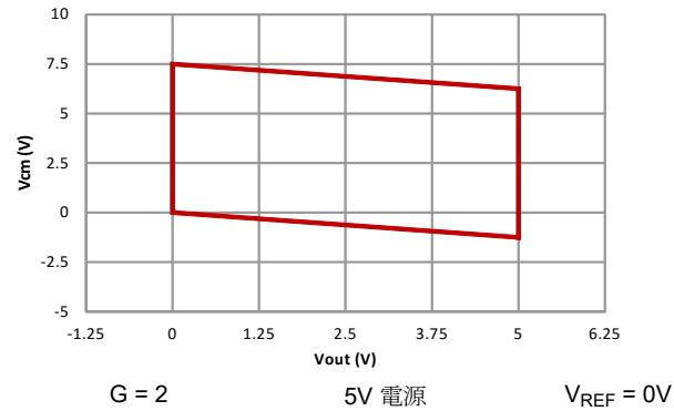
図 7-70. 入力同相電圧と出力電圧との関係
