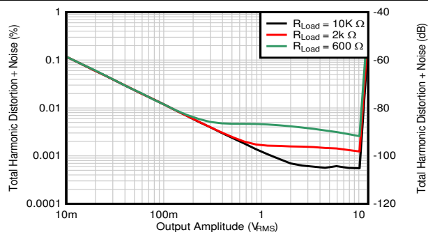
図 7-56. THD+N 比と出力振幅との関係
