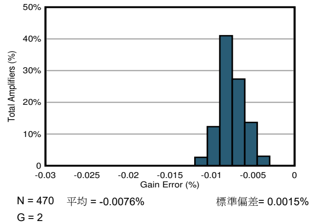
図 7-28. ゲイン誤差の標準的な分布
