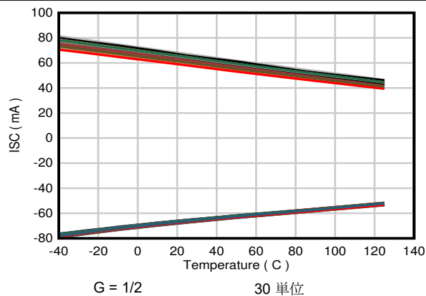
図 7-61. 短絡電流と温度との関係
