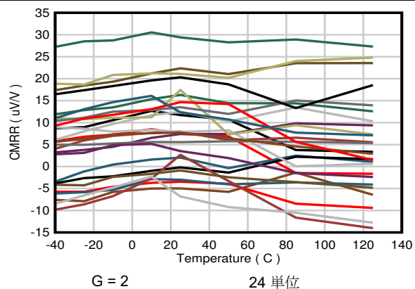
図 7-20. CMRR と温度との関係
