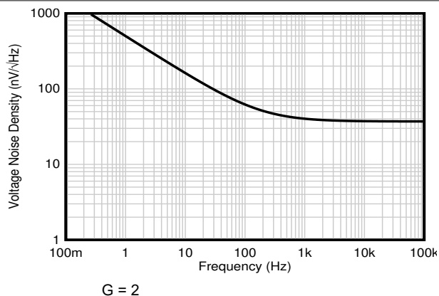
図 7-34. 電圧ノイズ・スペクトル密度と周波数との関係 (RTI)
