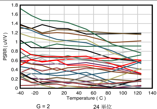
図 7-24. PSRR と温度との関係
