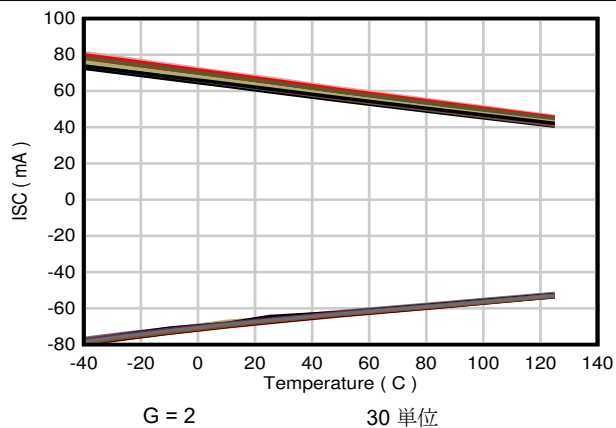
図 7-62. 短絡電流と温度との関係
