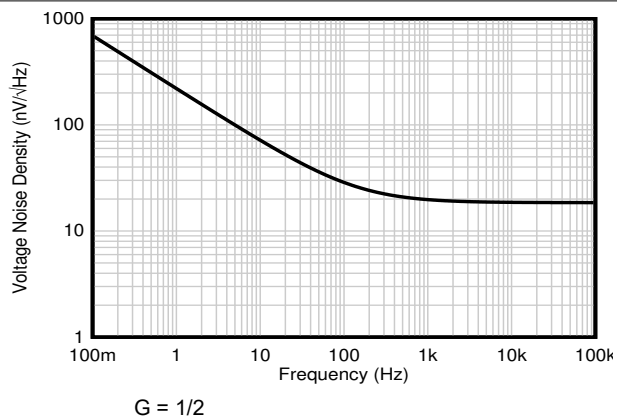
図 7-33. 電圧ノイズ・スペクトル密度と周波数との関係 (RTI)
