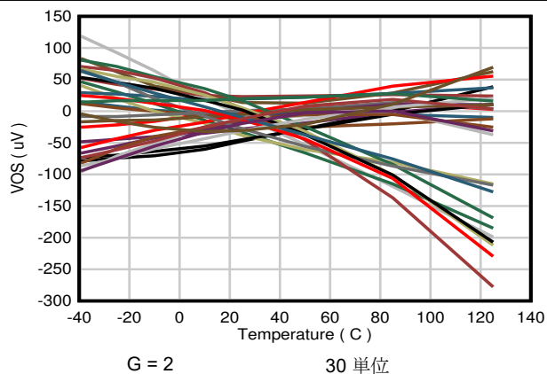
図 7-8. 出力オフセット電圧と温度との関係
