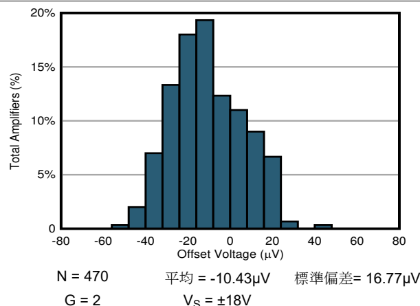
図 7-4. オフセット電圧の標準的な分布 (RTO)
