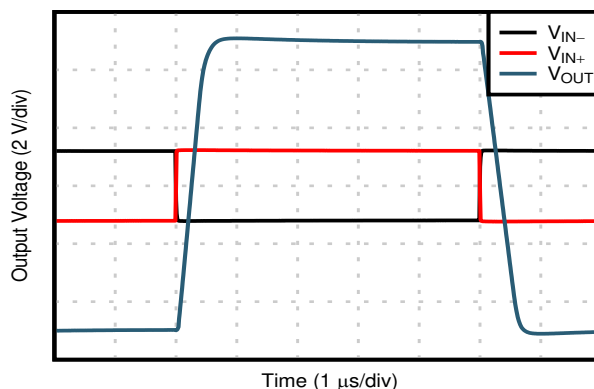
図 7-44. セットリング・タイム
