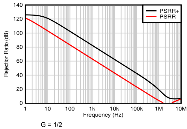
図 7-25. PSRR と周波数との関係 (RTI)
