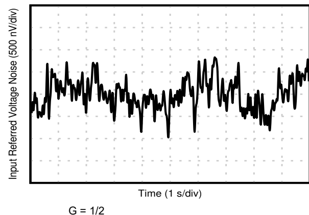
図 7-35. 0.1Hz~10Hz RTI 電圧ノイズ
