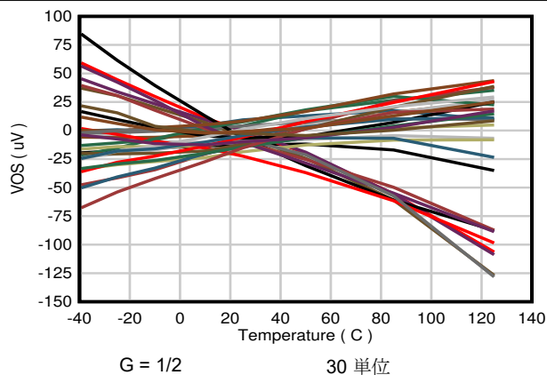
図 7-7. 出力オフセット電圧と温度との関係
