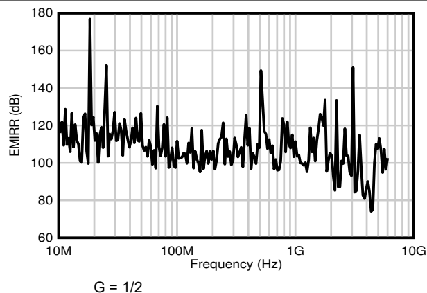
図 7-65. 同相 EMI 除去比
