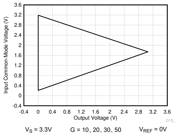
図 7-58. 入力同相電圧と出力電圧との関係
