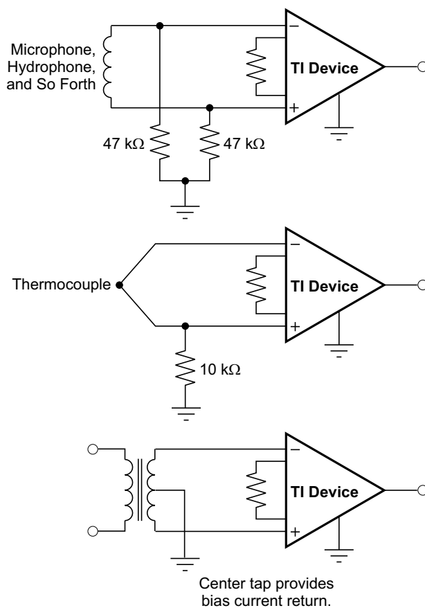
図 9-2. 入力同相電流パスの供給
