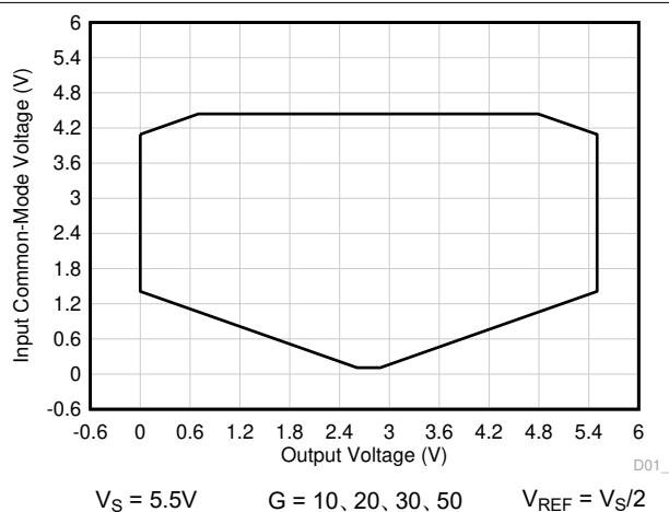
図 8-1. 入力同相電圧と出力電圧との関係 (高 CMRR 領域)
