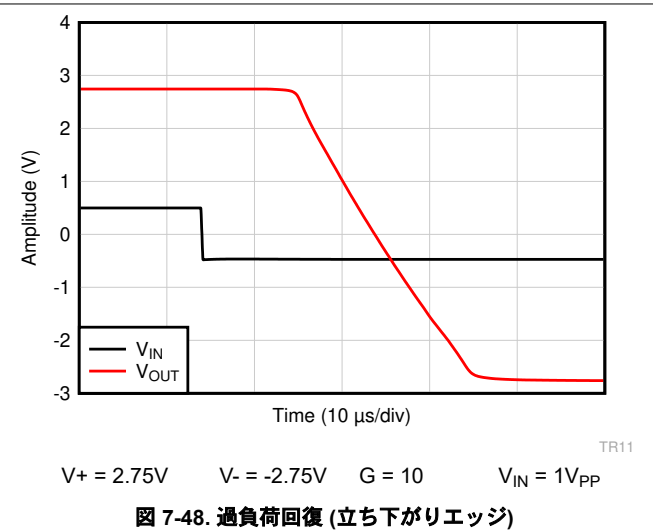
図 7-48. 過負荷回復 (立ち下がりエッジ)
