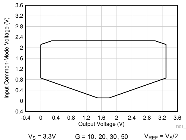
図 7-52. 入力同相電圧と出力電圧との関係 (高 CMRR 領域)
