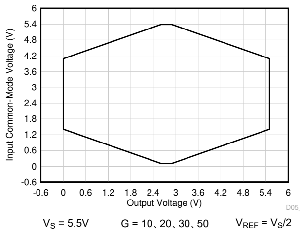
図 7-57. 入力同相電圧と出力電圧との関係
