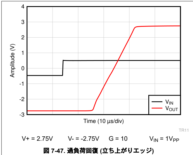
図 7-47. 過負荷回復 (立ち上がりエッジ)
