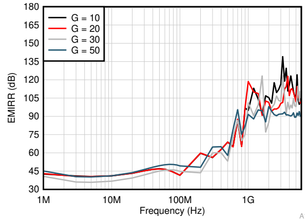
図 7-38. 非反転入力を基準とする電磁干渉除去比 (EMIRR+) と周波数との関係
