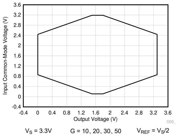
図 7-56. 入力同相電圧と出力電圧との関係
