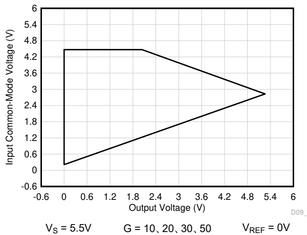
図 7-55. 入力同相電圧と出力電圧との関係 (高 CMRR 領域)
