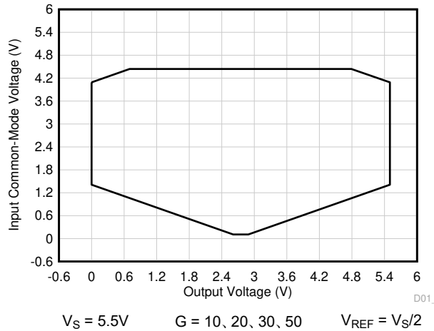
図 7-53. 入力同相電圧と出力電圧との関係 (高 CMRR 領域)
