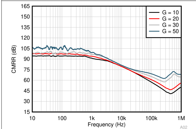
図 7-29. CMRR (入力換算) と周波数との関係
