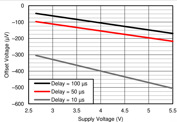
FIG 6-2. Input Offset Voltage
