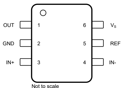
図 4-1. INA299 : DVB パッケージ 6 ピン SOT-23 上面図
