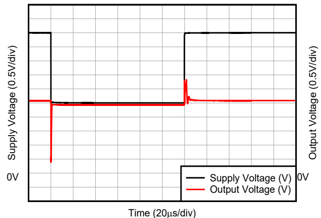
図 5-32. ブラウンアウトからの復帰
