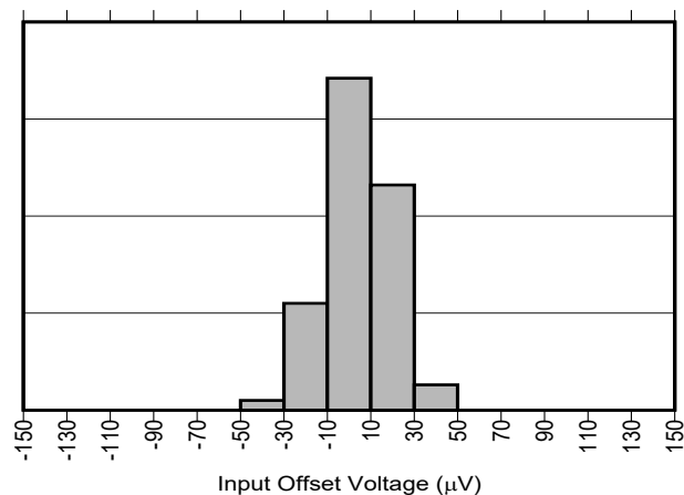
図 5-1. INA299 入力オフセット電圧の製品分布
