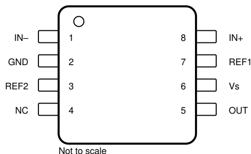
図 5-2. INA296x-Q1 : D および DGK パッケージ 8 ピン SOIC および 8 ピン VSSOP 上面図
