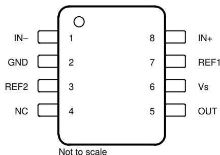
図 5-1. INA296x-Q1 : DDF パッケージ 8 ピン SOT-23 上面図
