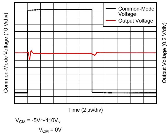
図 6-33. 同相電圧の高速過渡パルス
