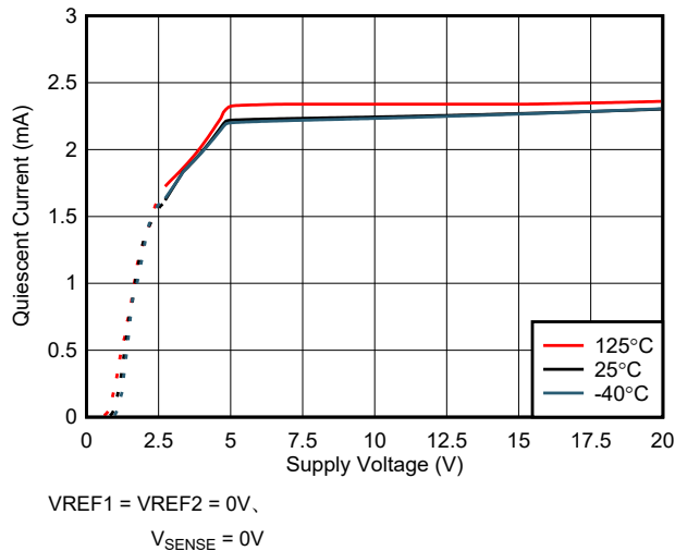
図 6-31. 静止電流と電源電圧との関係
