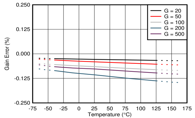
図 7-4. ゲイン誤差と温度との関係
