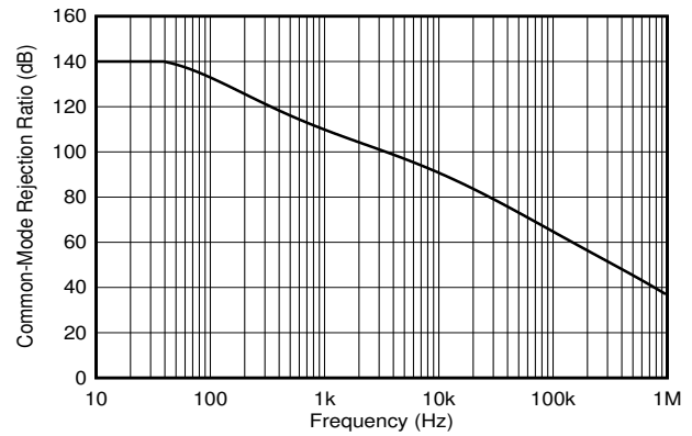
図 7-2. 同相除去比と周波数との関係
