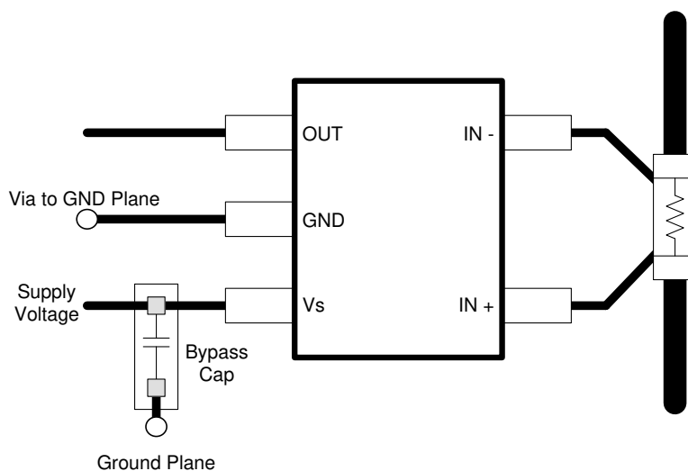
図 11-2. INA281B の推奨レイアウト
