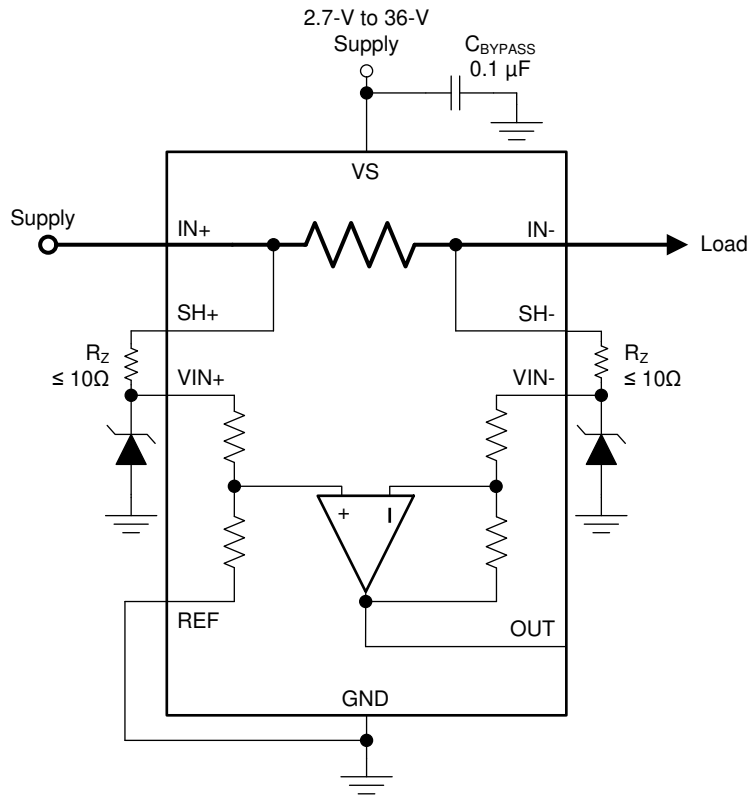
図 7-7. Device Transient Protection
