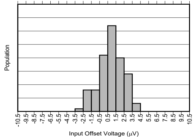
図 6-2. INA241A2-Q1 の入力オフセットの製品分布
