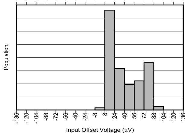
図 6-3. INA241A3-Q1 および INA241A4-Q1 の入力オフセットの製品分布
