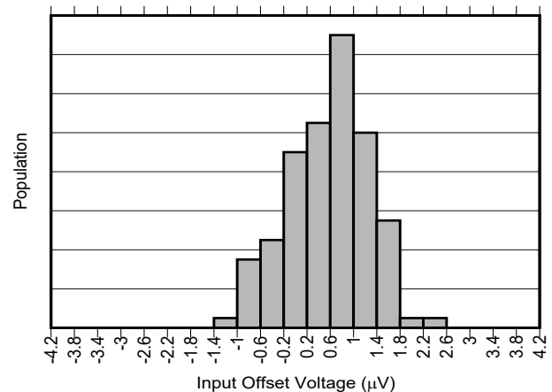
図 6-4. INA241A5-Q1 の入力オフセットの製品分布
