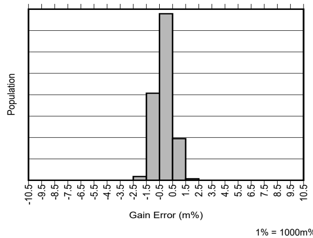
図 6-10. INA241A1-Q1、INA241A2-Q1、INA241A3-Q1 のゲイン誤差の製品分布 1% = 1000m%
