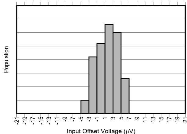
図 6-1. INA241A1-Q1 の入力オフセットの製造分布
