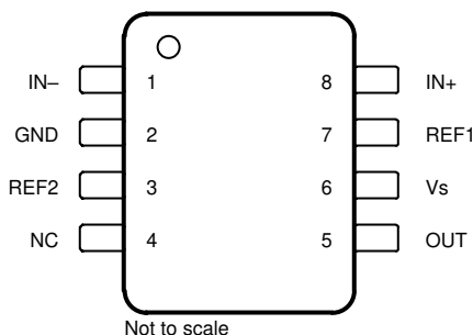
図 5-1. INA241x-Q1 : DDF パッケージ 8 ピン SOT-23 図 5-2. INA241x-Q1:D および DGK パッケージ 8 ピン SOIC および 8 ピン VSSOP 上面図
