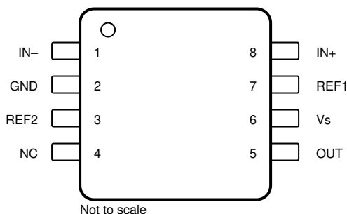
図 5-1. INA241x-Q1 : DDF パッケージ 8 ピン SOT-23 図 5-2. INA241x-Q1:D および DGK パッケージ 8 ピン SOIC および 8 ピン VSSOP 上面図
