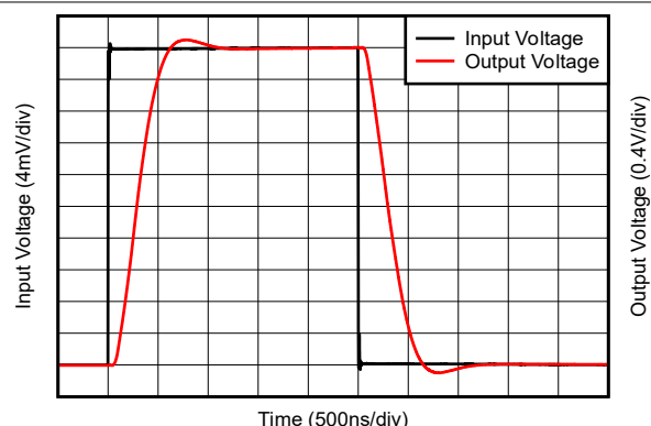
図 6-35. 大ステップ応答
