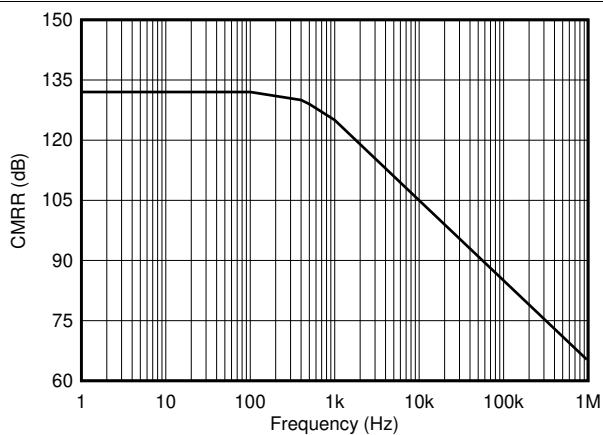
図 7-12. 同相除去比と周波数との関係
