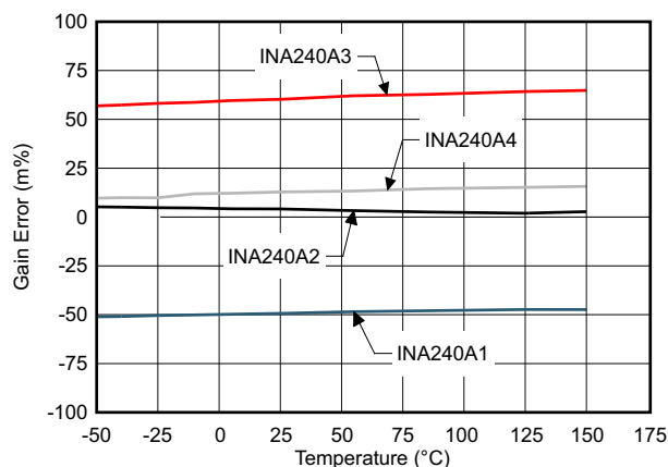
図 7-9. ゲイン誤差と温度との関係
