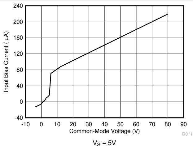
図 7-14. 入力バイアス電流と同相電圧との関係
