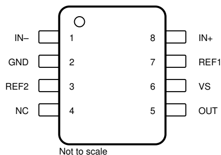
図 6-2. INA240-Q1 D パッケージ 8 ピン SOIC 上面図
