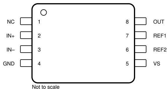
図 6-1. INA240-Q1 PW パッケージ 8 ピン TSSOP 上
