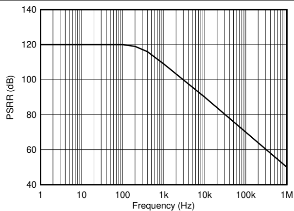
図 7-11. 電源除去比と周波数との関係
