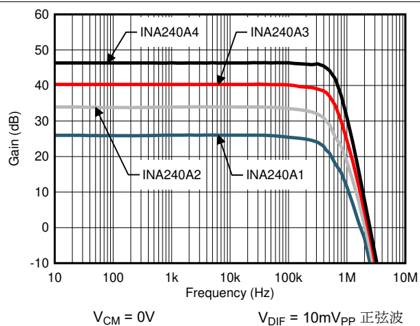
図 7-10. ゲインと周波数との関係
