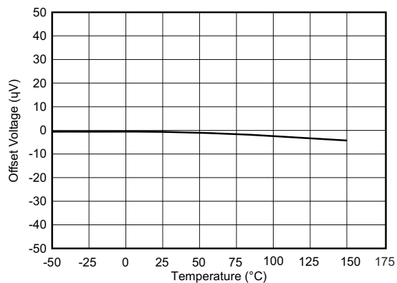
図 7-2. オフセット電圧と温度との関係
